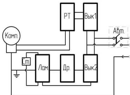
Рис.4. Схема среднетемпературной витрины с электронным блоком управления.
